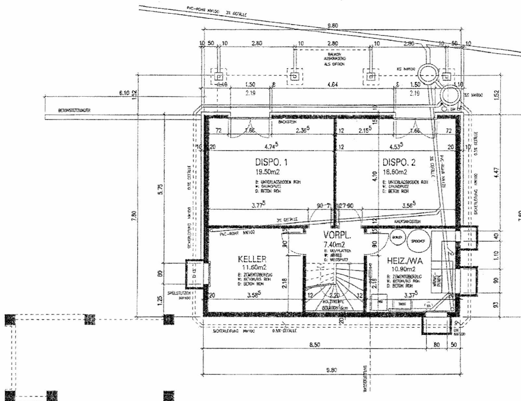
UNTERGESCHOSS 1:100
